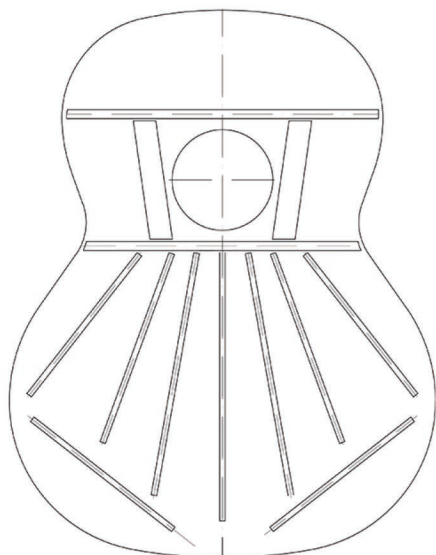
M2 Bracing Pattern Verwendet bei: Solea
