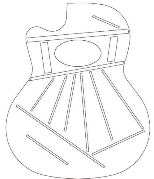
M6 Bracing Pattern Verwendet bei
