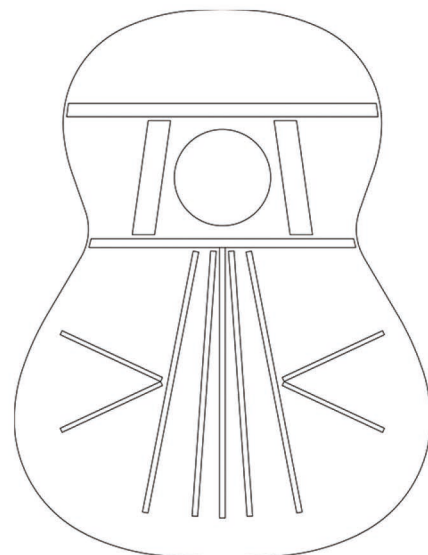
M7 Bracing Pattern Verwendet bei 90th Anniversary
